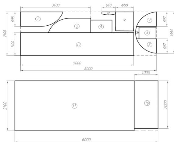
Рис.1 Сема раскроя поликарбоната
