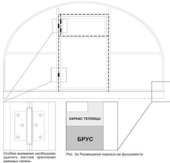
Рис.3 Схема вырезов для двери и форточки
