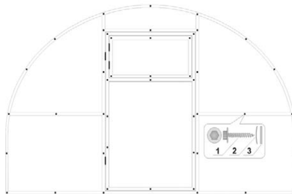
1. Саморез, 2. Шайба, 3. Резиновая прокладка
